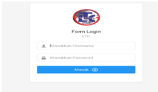
Gambar 3. Menu Login
